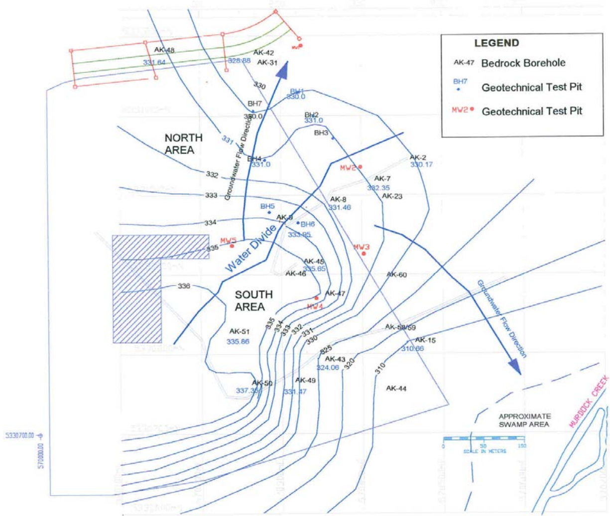
Figure 4-7 Groundwater equipotential map.
